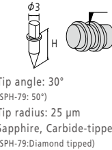
Cone stylus
