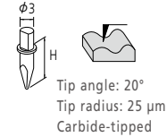
Cone stylus
