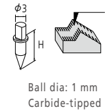
Ball stylus
